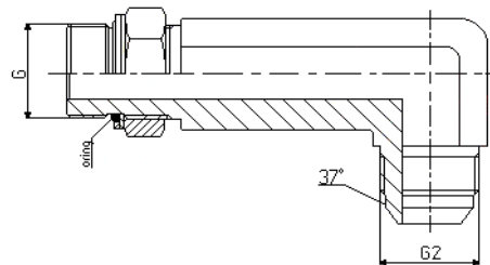
JIC XWESVGUNF / UNF
