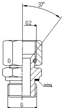
JIC EGE UNF / UNF
