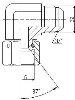
JIX XEW UNF / UNF
