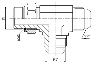
JIC XETP M / UNF
