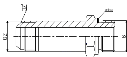
JIC XESVGBSP / UNF
