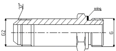
JIC XESVGUNF / UNF
