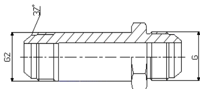
JIX XEW UNF / UNF
