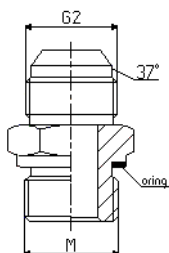
JIC XGE M / UNF
